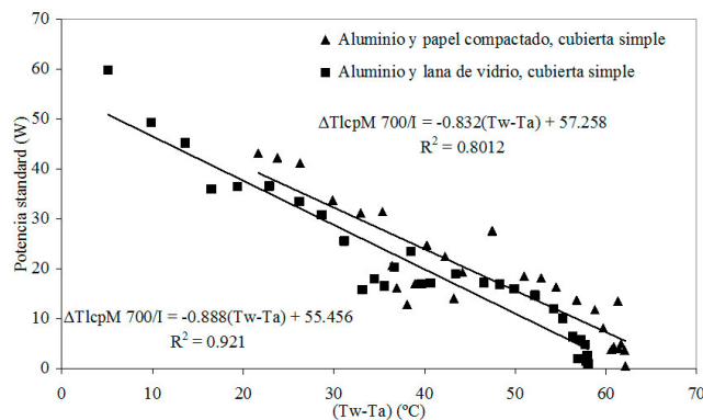
Figura 3. Ajuste lineal entre la potencia standard y la diferencia de temperatura del líquido de prueba
