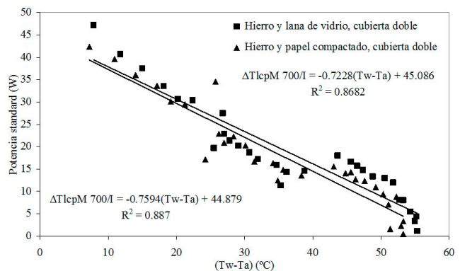
Figura 3. Ajuste lineal entre la potencia standard y la diferencia de temperatura del líquido de prueba
