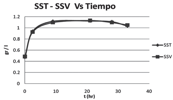
Figura 8. Comportamiento de los SST y SSV frente a tiempo
