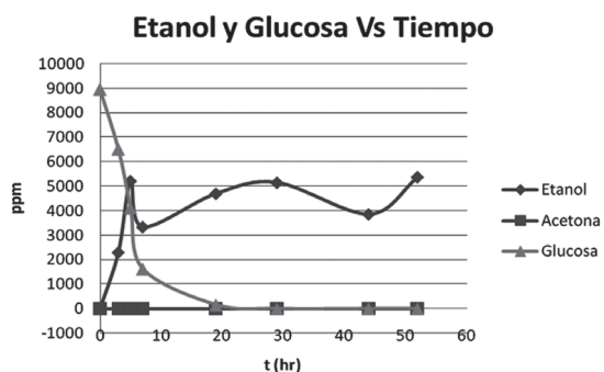
Figura 5. Comportamiento del etanol producido y la glucosa frente a tiempo
