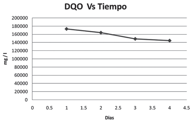
Figura 3. Variación DQO frente a Tiempo
