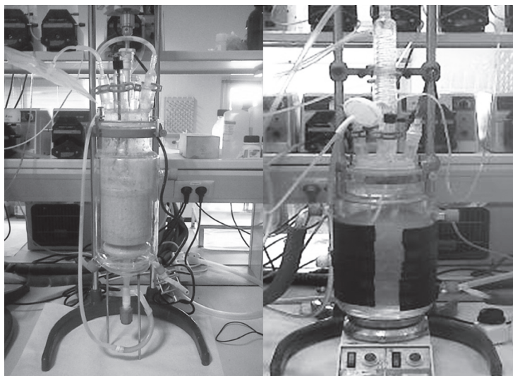
Imágenes 1 y 2. Pruebas y puesta en marcha del biorreactor para el desarrollo de las fases de fermentación de la FORSU. Laboratorios UCLM – Ciudad Real, España.
