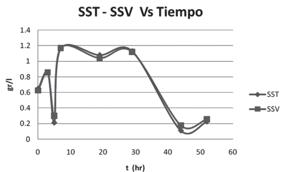
Figura 6. Comportamiento de los SST y SSV frente a tiempo
