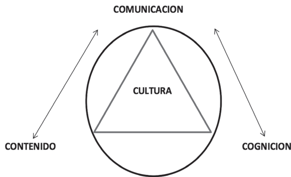
Figura 1. Diagrama AICLE
